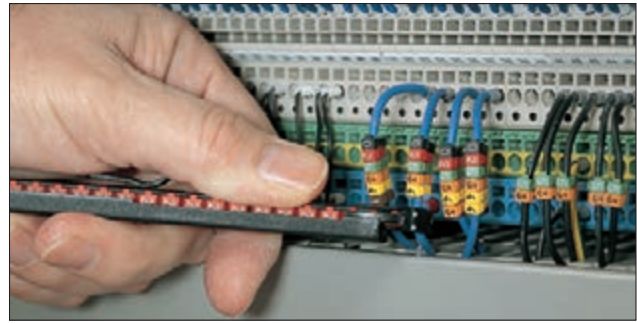
WIC-Markierer eignen sich besonders für die Kennzeichnung nach der Montage.
