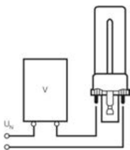
Schaltplan
