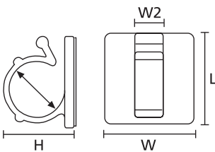
Befestigungssockel RA3-18
