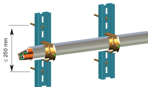
Verlegeabstand: ≤ 1.200 mm
