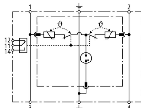
Prinzip Schaltbild DR M 2P 30 FM
