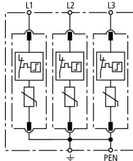
Prinzipschaltbild DG M WE 600
